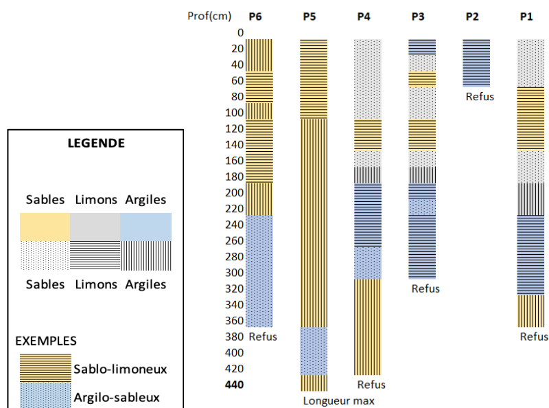
Figure 13. Strates sédimentaires traversées par les prélèvements à la tarière
