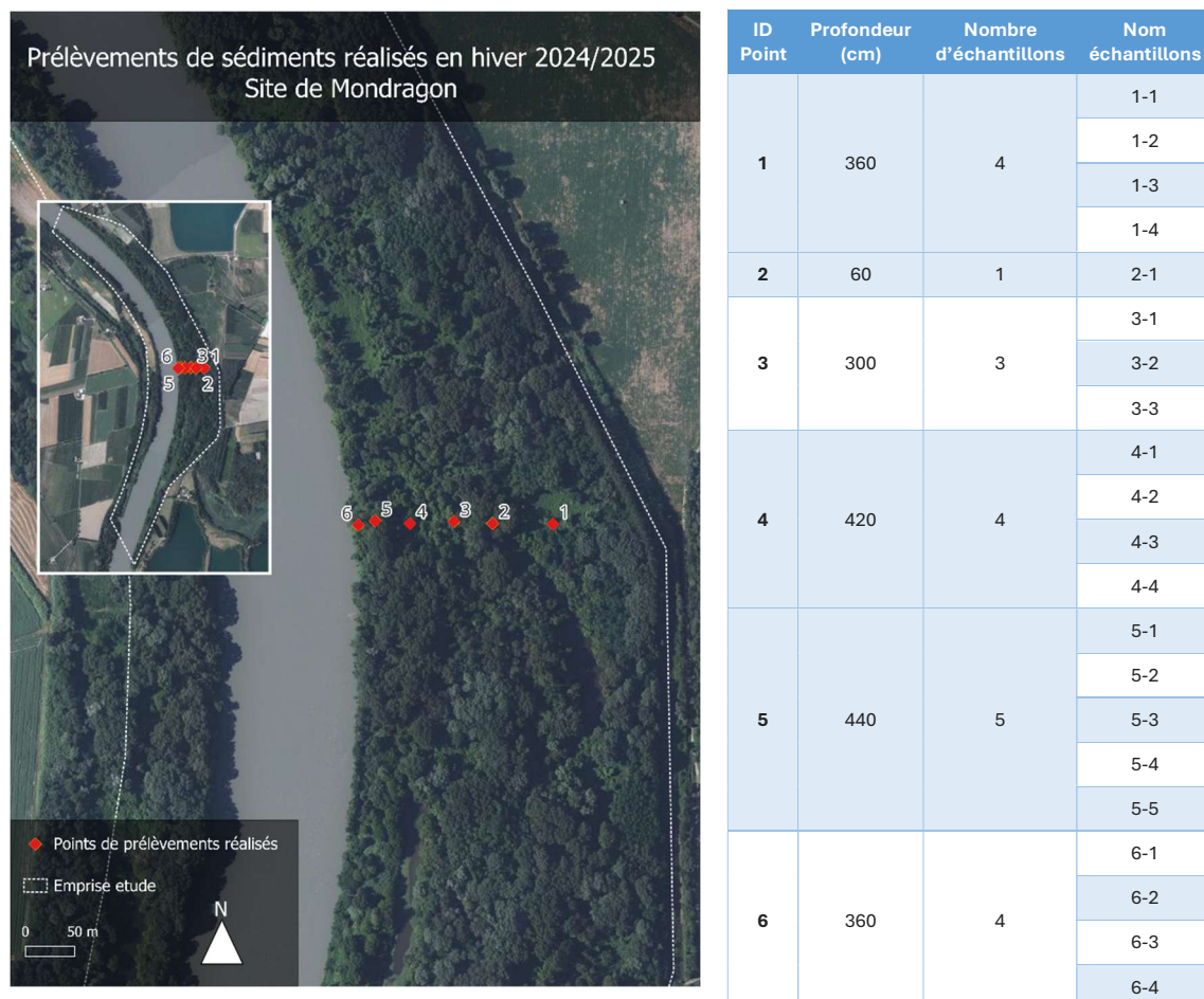
Figure 15 : Localisation du profil et des sondages. Tableau récapitulatif des prélèvements effectués par sondage et par tranche de sol (GEOPEKA)
