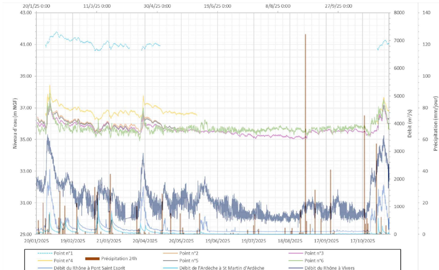
Figure 9 : Graphique compilé des mesures de niveaux d'eau des 6 sondes et des données hydrologiques et pluviométriques (GEOTHER)
